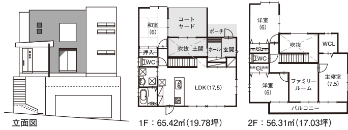
C号地 立面図・間取り図
